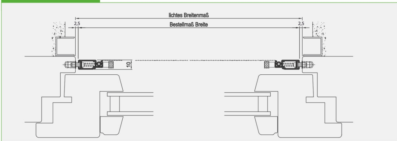
Horizontalschnitt M = 1: 2.5
